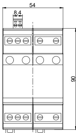
Габаритные размеры
