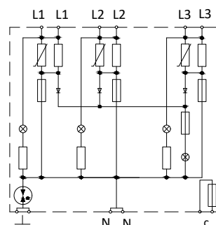
Принципиальная схема
